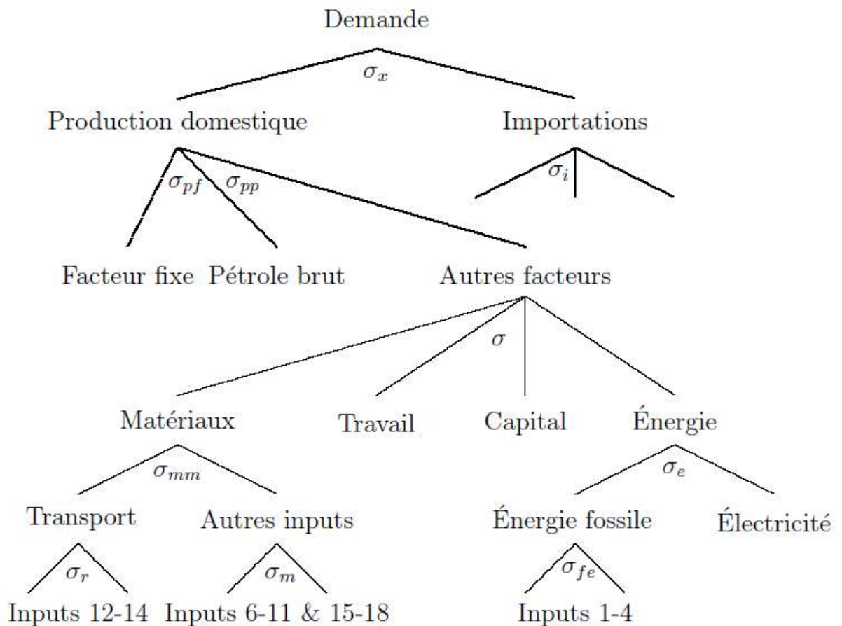
Figure 1: Structure de la production dans GEMINI-E3
