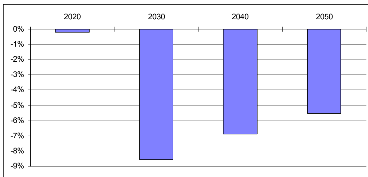
Figure 4 : Baisse en pourcentage des émissions de CO 2 Tunisiennes
