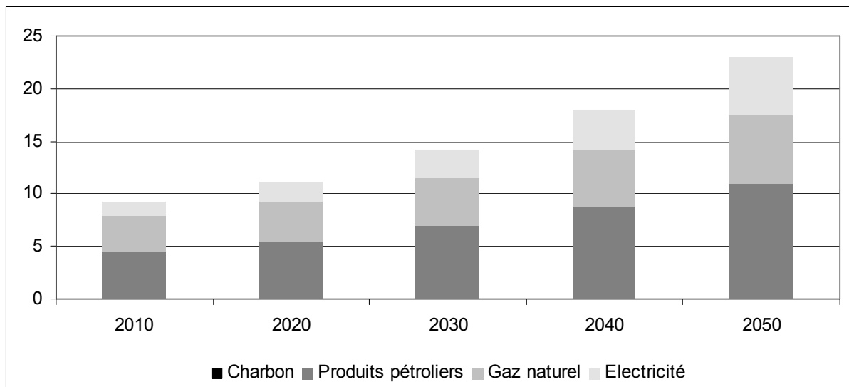
Figure 1: Consommation d'énergie en Tunisie en Mtep
